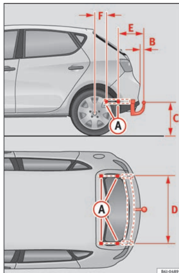
Fig. 153 IBIZA/IBIZA SC : points de fixation du dispositif de remorquage.
