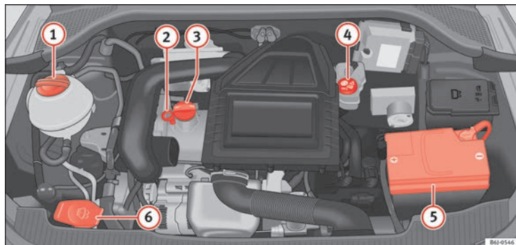
Fig. 154 Figure d'exemple de la position des éléments.
