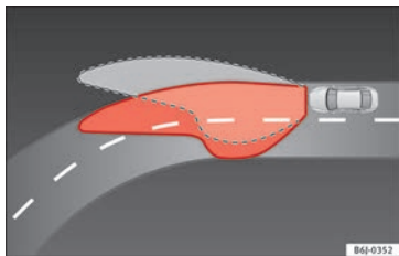
Fig. 118 Éclairage du virage à l'aide des phares autodirectionnels.
