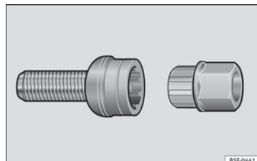
Fig. 57 Boulon antivol de roue avec capuchon et adaptateur.
