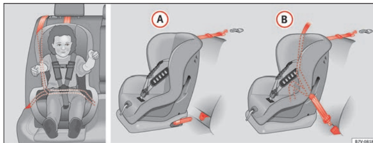
Fig. 22 Sur les sièges arrière : installations possibles d'un siège pour enfants.
