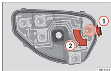
Fig. 99 Remplacement des ampoules des feux arrière.
