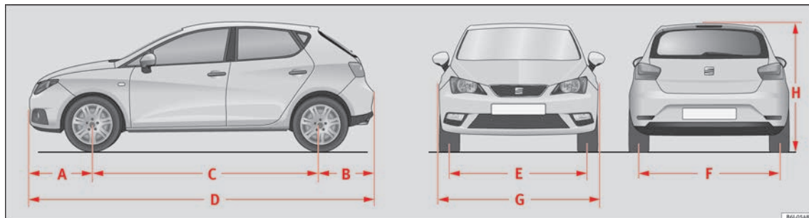
Fig. 162 Dimensions
