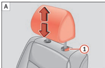
Fig. 153 Montage de l'appuie-tête de la deuxième ou troisième rangée de sièges.
