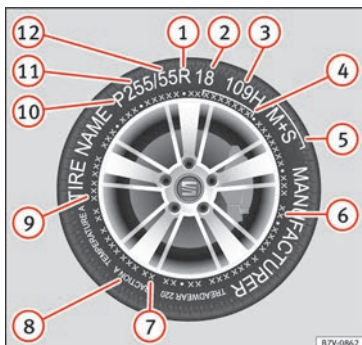
Fig. 253 Inscription universelle sur les pneus.
