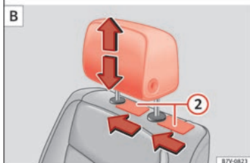
Fig. 152 A : Montage des appuie-tête sans possibilité de réglage en longueur ; B : Montage des appuie-tête avec possibilité de réglage en longueur.
