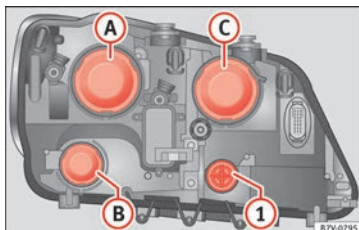
Fig. 105 Dans le compartiment moteur : revêtements dans le phare gauche. A feux de croisement, B feux de jour et C feux de route et feux de position.
