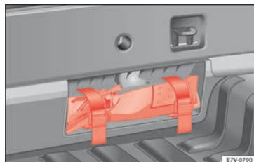
Fig. 99 Dans le coffre, vu depuis l'intérieur du véhicule : outillage de bord dans une cavité située dans la zone du porte-serrure.
