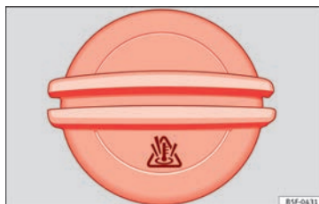
Fig. 56 Compartiment-moteur : bouchon du vase d'expansion du liquide de refroidissement.
