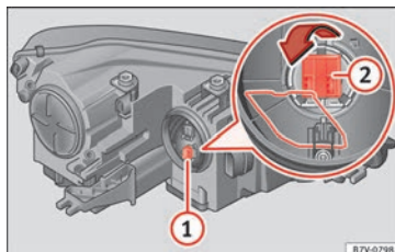
Fig. 107 Dans le compartiment moteur : cache du clignotant.
