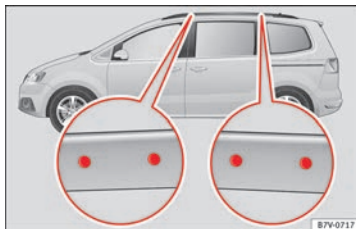
Fig. 174 Points de fixation des supports standard et de la galerie porte-bagages du toit.
