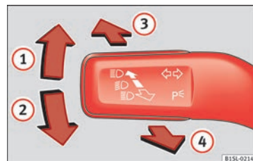
Fig. 41 Lever des clignotants et des feux de route.
