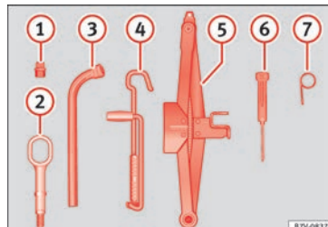
Fig. 64 Dans le coffre à bagages, sous le revêtement du plancher de chargement : outillage de bord.
