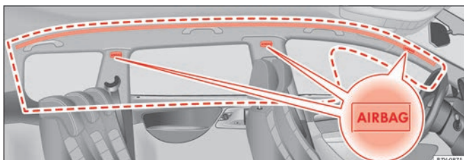
Fig. 32 Sur le côté gauche du véhicule : emplacement et champ d'action de l'airbag de tête.
