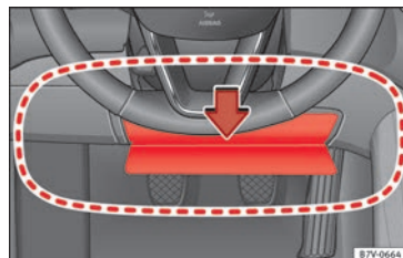
Fig. 29 Côté conducteur : rayon d'action de l'airbag de genoux.
