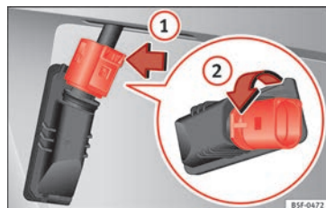
Fig. 116 Feu de plaque d'immatriculation : Démontez le porte-ampoule.
