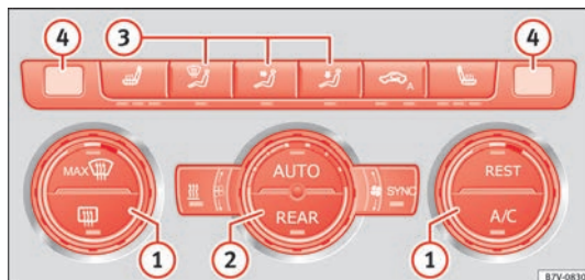
Fig. 52 Détail de la console centrale : commandes du Climatronic.
