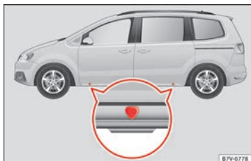
Fig. 69 Points de prise du cric.
