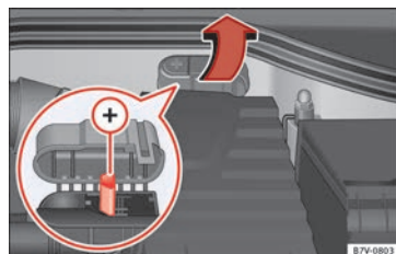
Fig. 74 Dans le compartiment moteur : pôle positif d'aide au démarrage (+).
