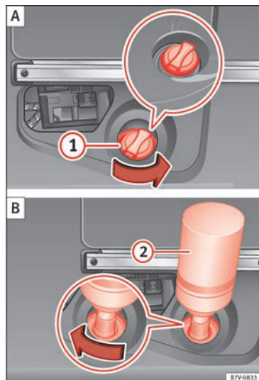
Fig. 237 Réservoir d'AdBlue avec bouchon de fermeture de la goulotte de remplissage et un bidon pour rajouter du liquide.
